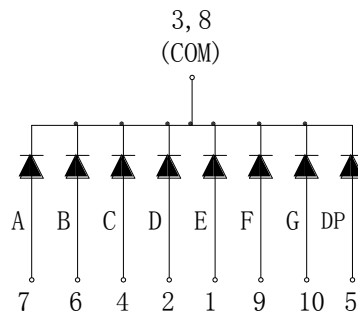
DL1-1001CWB-1C
