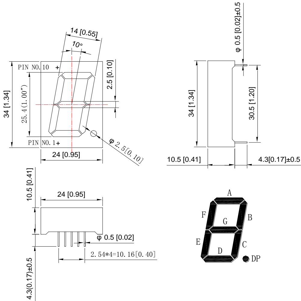
DL1-1001AWB-1C
