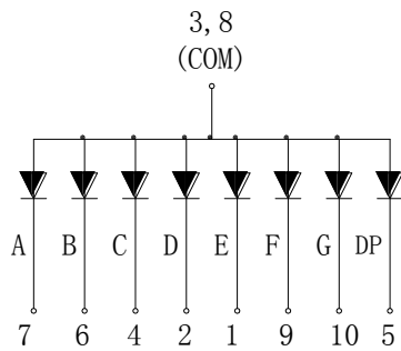
DL1-1001AWB-1C
